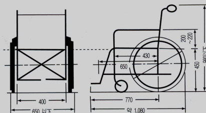
● 휠체어 배면 및 측면도
